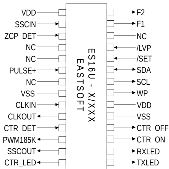
28-引脚封装图
