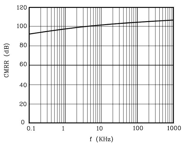
Fig. 5 CMRR-f
