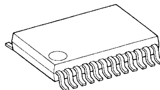
SSOP24-P-300-0.65A
