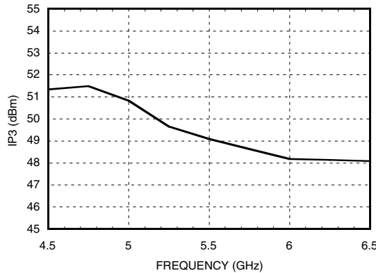
Input IP3 *
