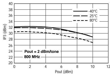
OIP3 vs. Pout
