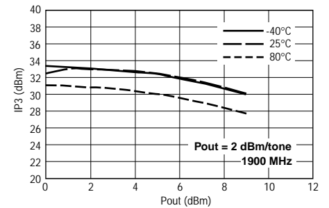
OIP3 vs. Pout
