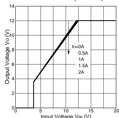
Rise Characteristics(SI-3120J)
