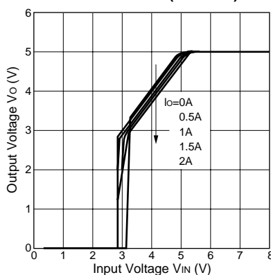
Rise Characteristics(SI-3050J)
