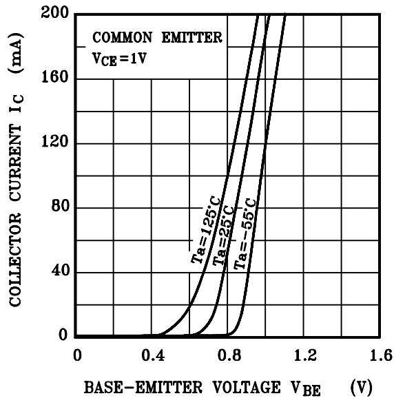
I_C - V_{BE}
