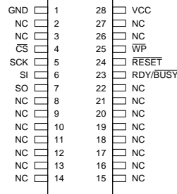
SOIC
