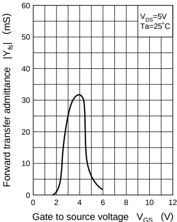
|Y_{fs}| - V_{GS}
