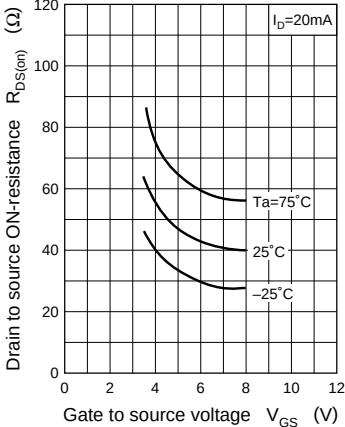
R_{DS(on)} - V_{GS}
