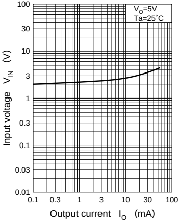
V_{IN} - I_O
