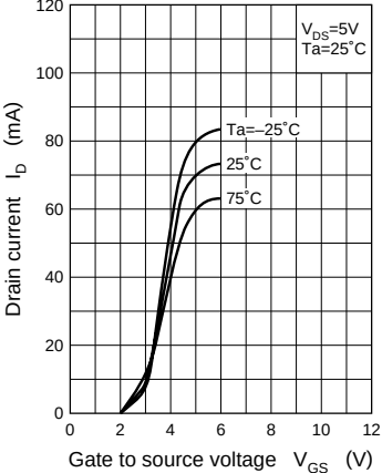
I_D - V_{GS}
